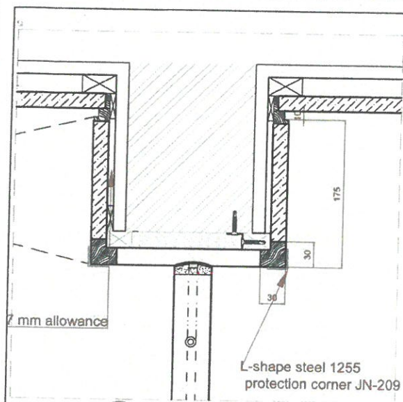
D1 Junction details
