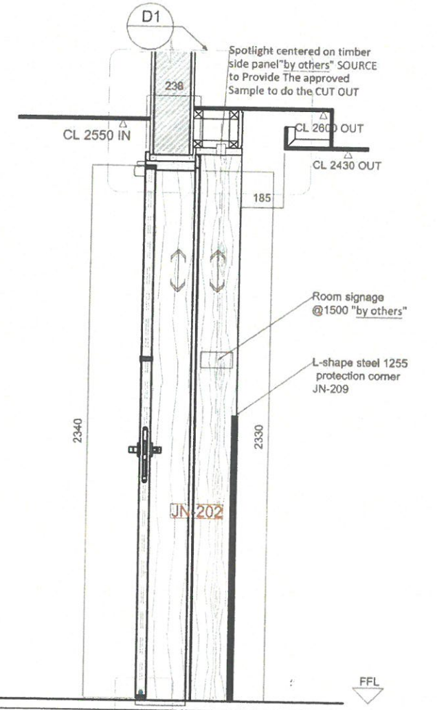
D2 Section
